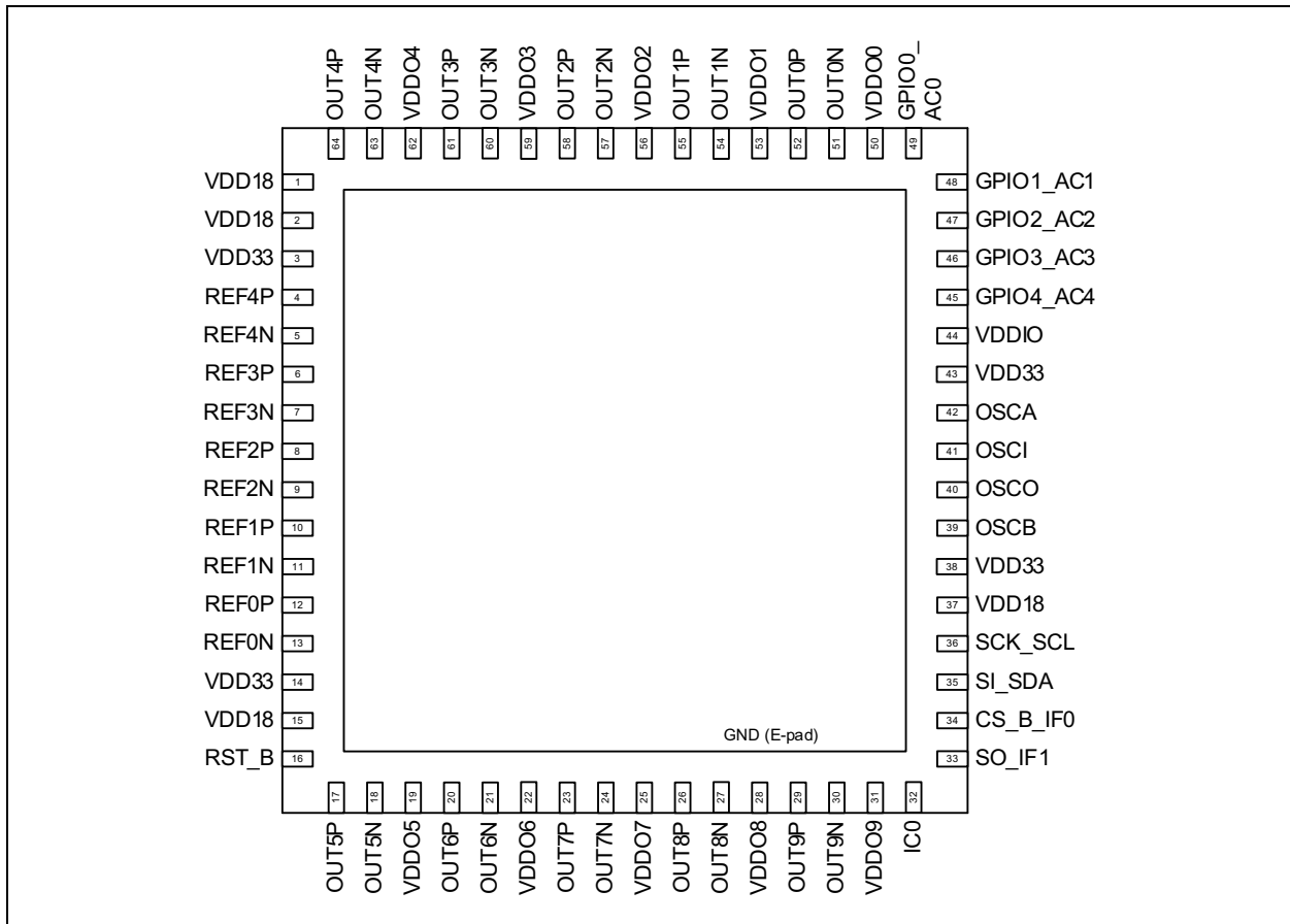
図 4-1: ZL30631、ZL30632、ZL30633、ZL30634、ZL30635 向け 64 ピン 9 mm x 9 mm VQFN (0.5 mm ピッチ)
