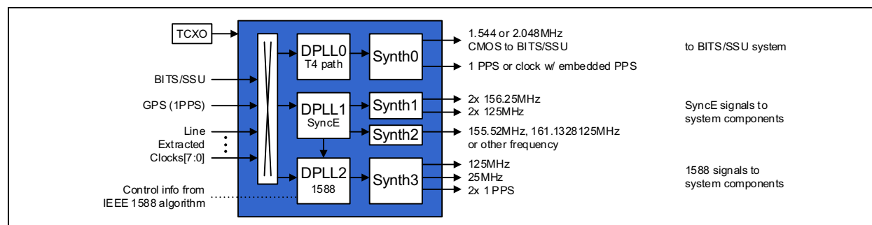
図 2-1: シンクロナス Ethernet と IEEE 1588 の標準時刻アプリケーション
